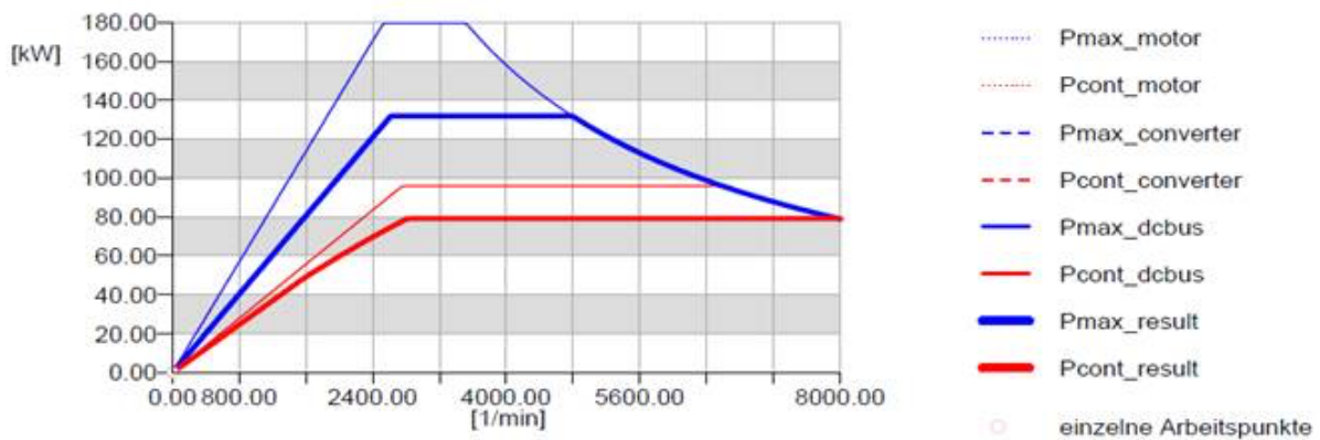
Drehzahl – Leistung - Diagramm
